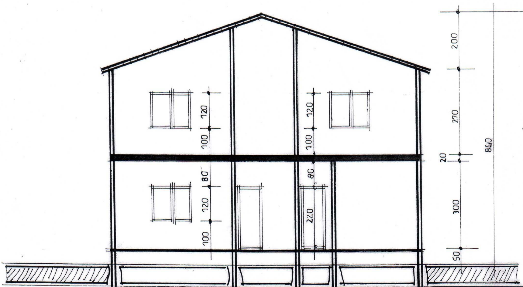
— · COUPE AA · —
