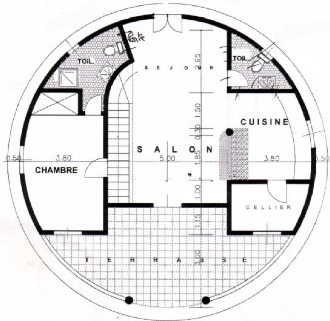
Plan REZ de CHAUSSEE
